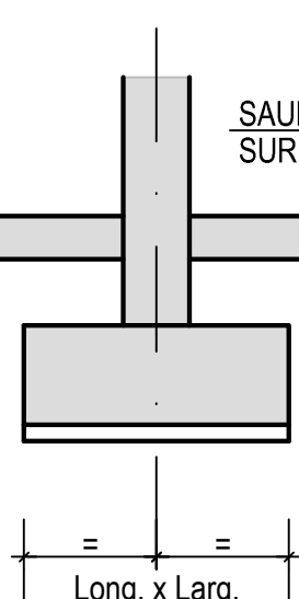
COUPES TYPES SEMELLES ISOLEES
